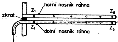
Obr. 6. Konstrukce i napájení antény LPD i LPDV zjednoduší dvoudílné nosné ráhno, které zároveň působí jako symetizační obvod
